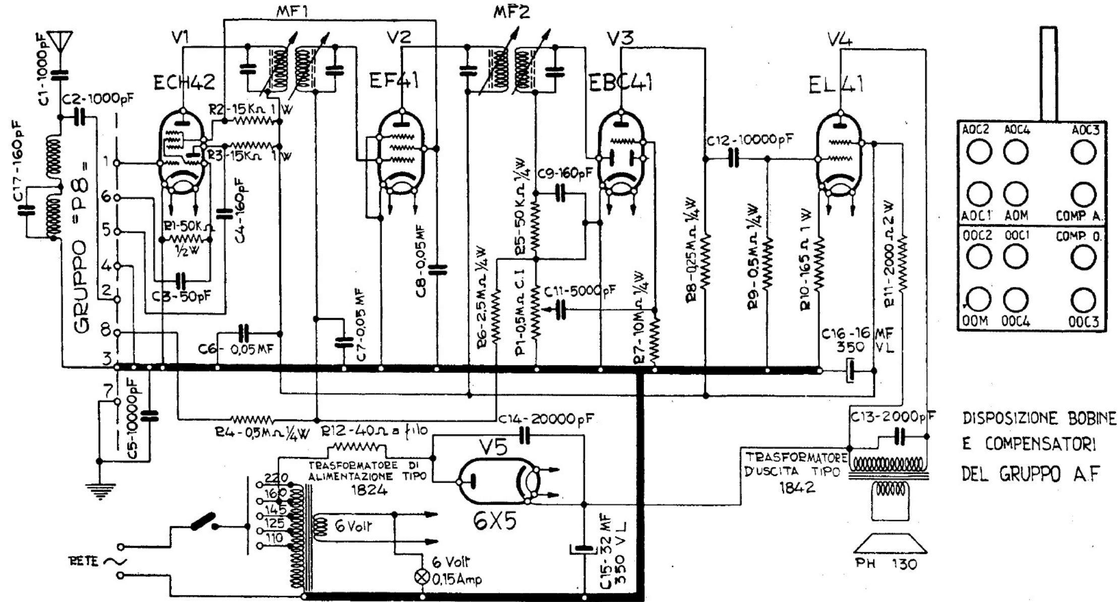
NOVA RADIO - Mod. G 2 - Funziona con gruppo P8. Media frequenza 465 kc. Funziona con valvole rimlock. Tensione anodica massima 155 volt; corrente anodica massima 48 mA.
